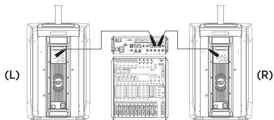
2 X EVOX J8 И ВНЕШНИЙ МИКСЕР (стерео)
