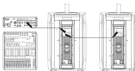
EVOX JMIX8 + EVOX J8 (стерео)
